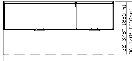
FPT-67 TOP
