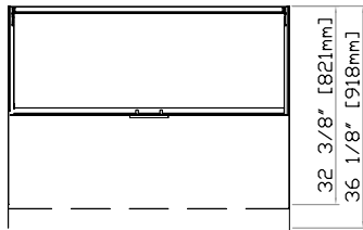
FPT-46 TOP
